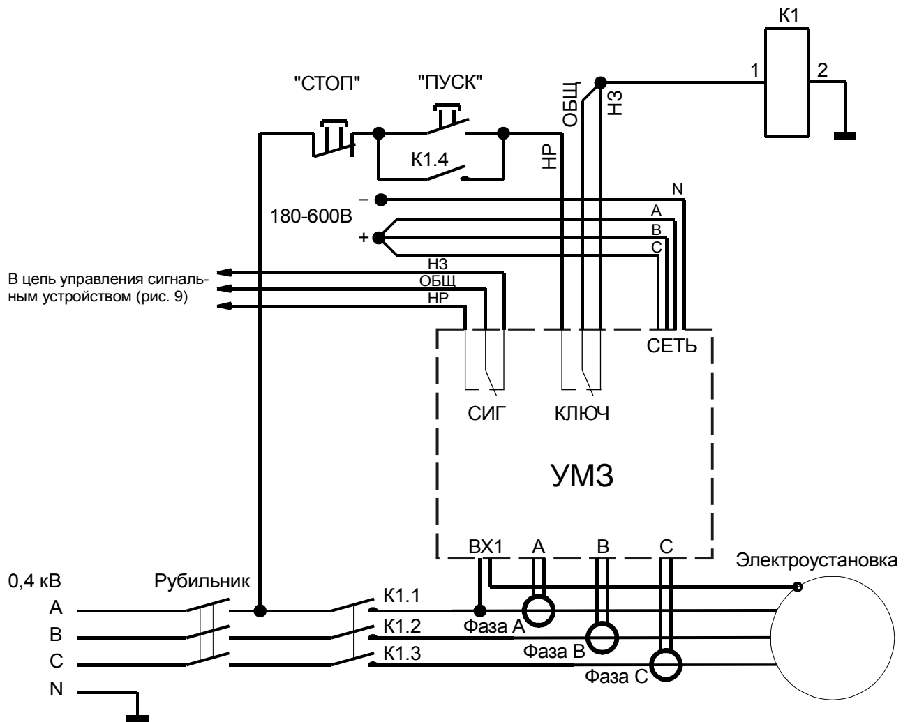
Рисунок 6. - Подключение устройства УМЗ в схему управления контактора переменного тока с предотвращением самозапуска при восстановлении питания. Питание УМЗ от источника постоянного тока.
