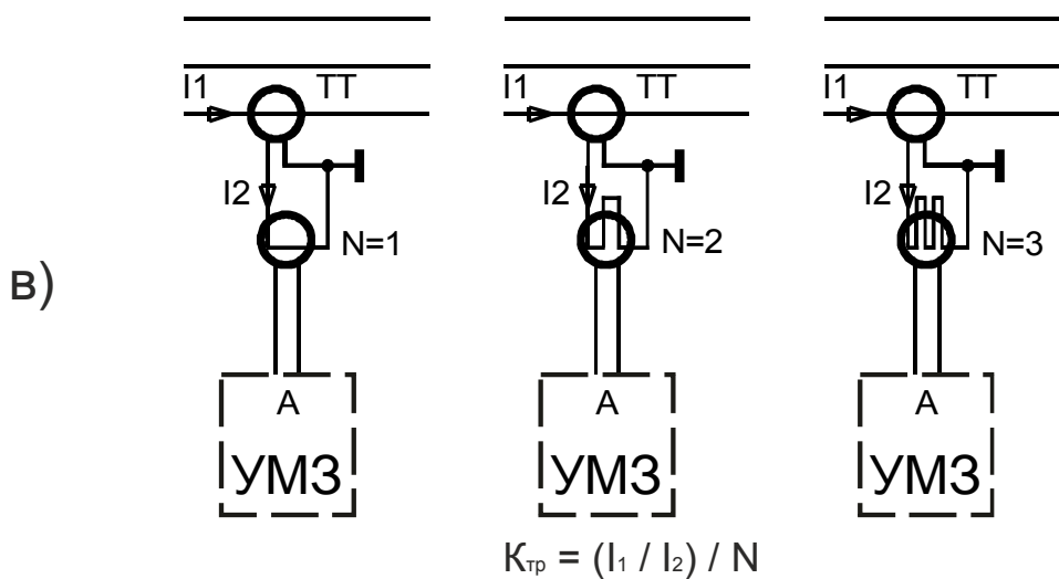
Рисунок 11. - Варианты схем косвенного подключения датчиков тока устройства УМЗ-10.
