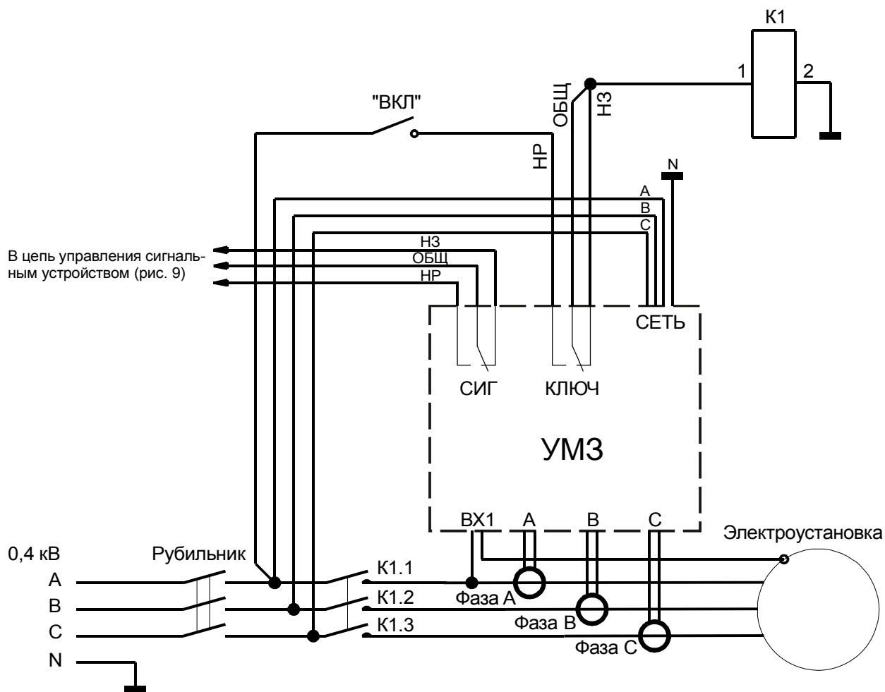
Рисунок 4. - Подключение устройства УМЗ в схему управления контактора переменного тока с самозапуском при восстановлении питания. Питание УМЗ от трех фаз. Примечание. При использовании контактора с катушкой на 380 В вывод 2 катушки K1 подключается к фазе В или С.
