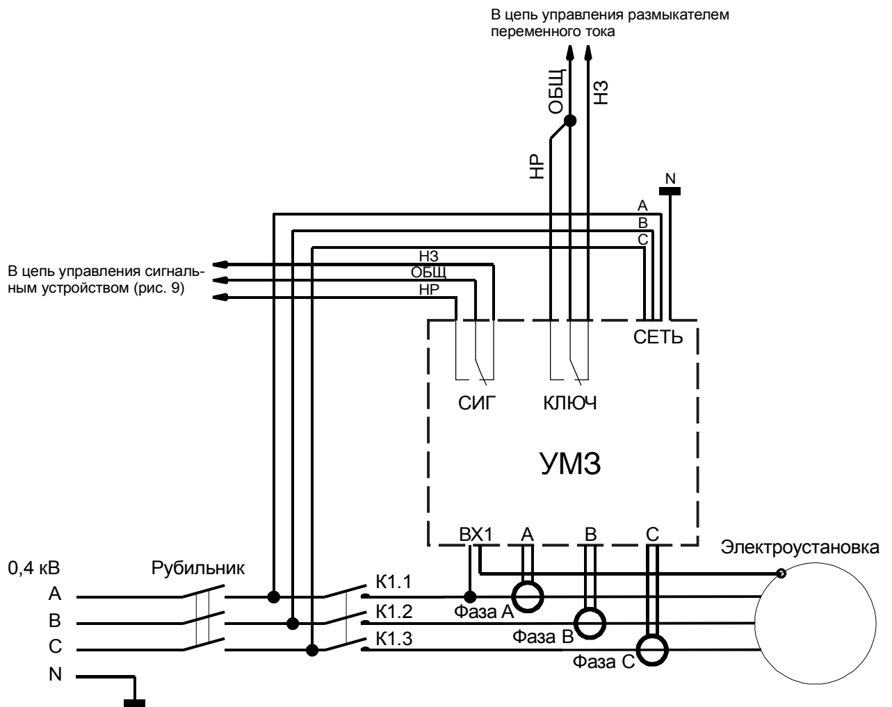
Рисунок 7. - Подключение устройства УМЗ в схему управления размыкателем переменного тока. Питание УМЗ от трех фаз.
