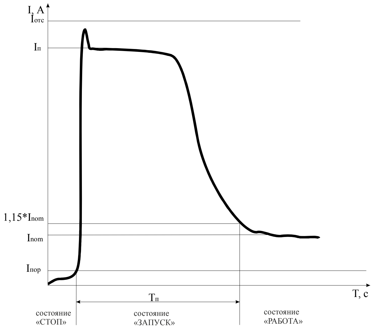
Рисунок 10. - Пусковая характеристика электроустановки и признаки изменения состояний устройства УМЗ. ( I_{пор} – нижняя граница диапазона контролируемых фазных токов (см. п. 2.2.1), I_{п} – пусковой ток электроустановки, T_{п} - время пуска электроустановки).
